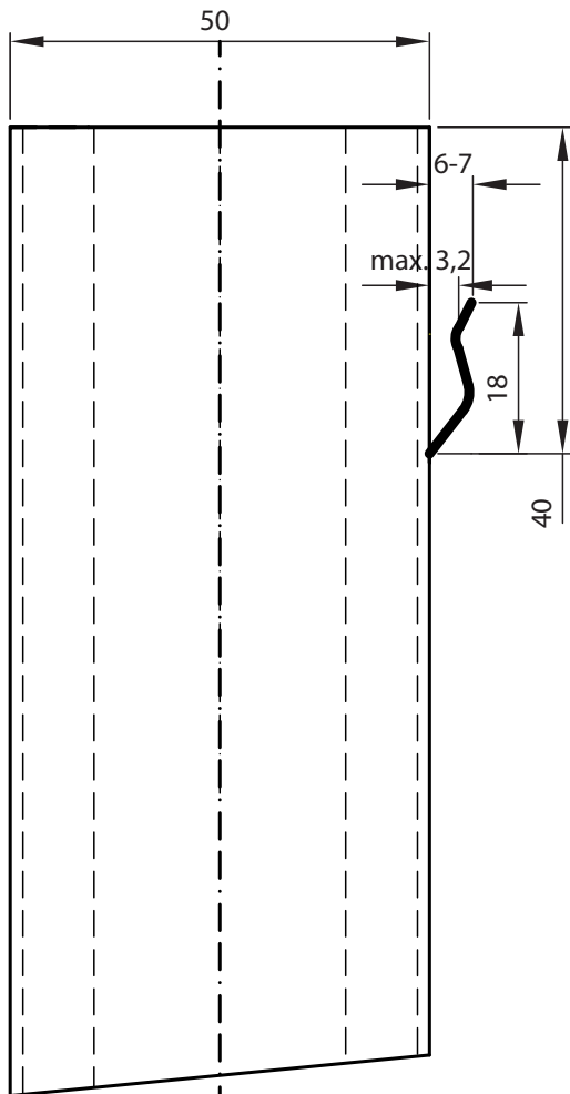
ŘEZ PROFILEM SLOUPKU
